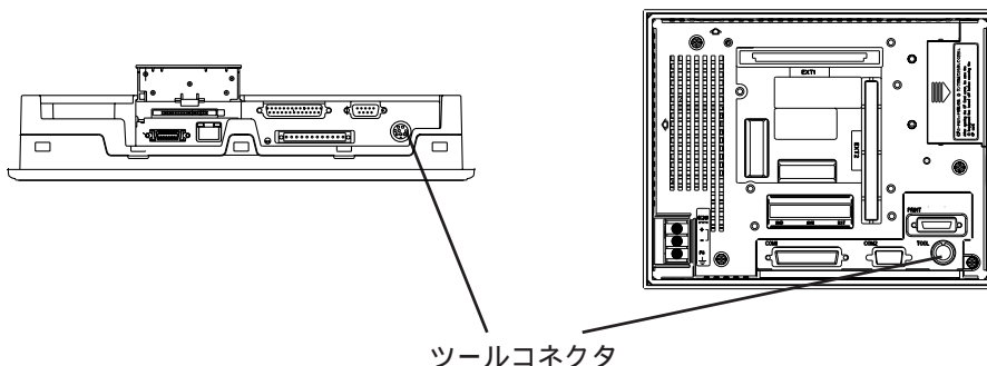
GP-2500T/GP-2600T 底面図
