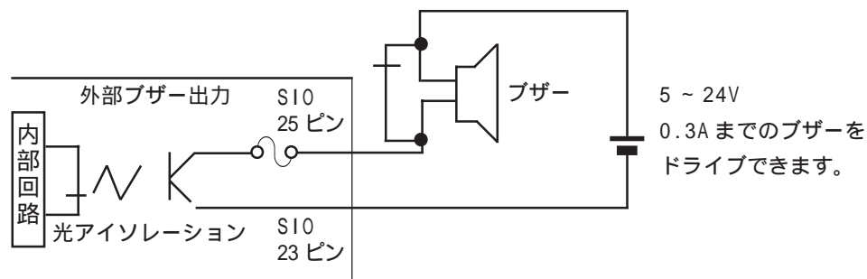
GP-377R シリーズ 本体内部
