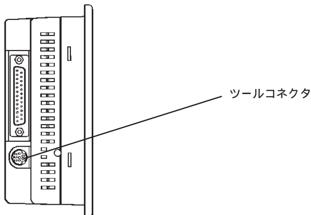
側面図
