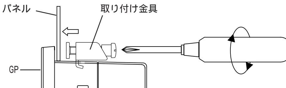
上面図
