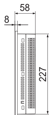
側面図
