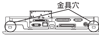
下面図
