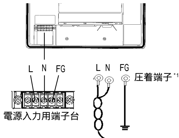
背面図
