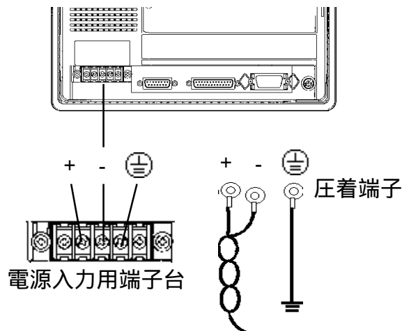
背面図
