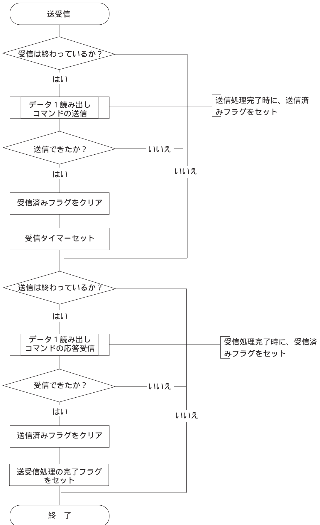
送受信関数1のフローチャート
