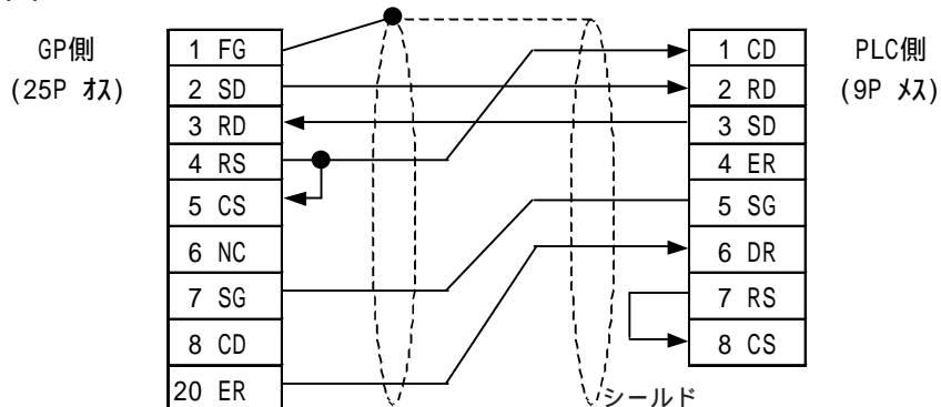
< 結線図 6 > RS-232C
