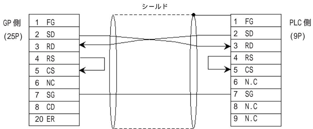
< 結線図 7 > RS-232C
