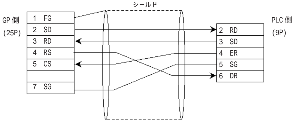
< 結線図 6 > RS-232C
