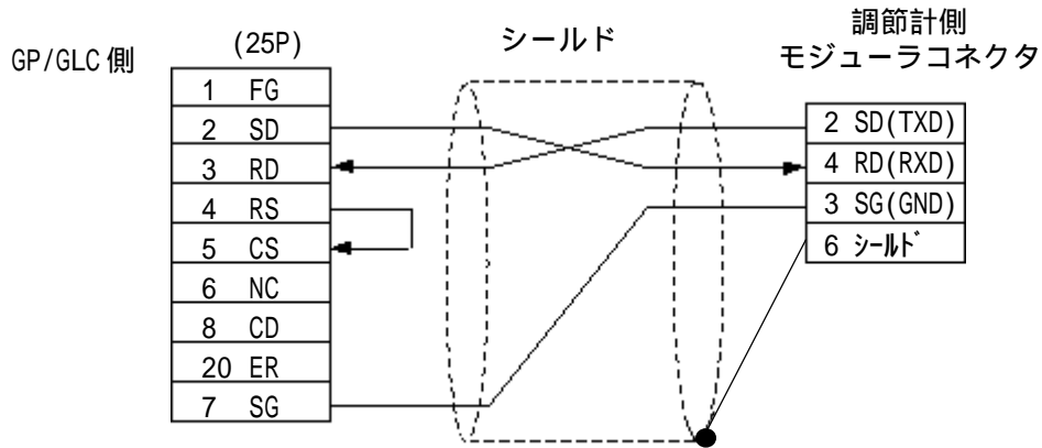
< 結線図 1 > 1:1 RS-232C
