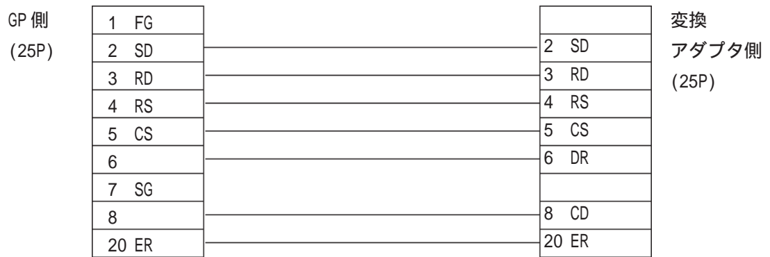
< 結線図 4 > RS-232C
