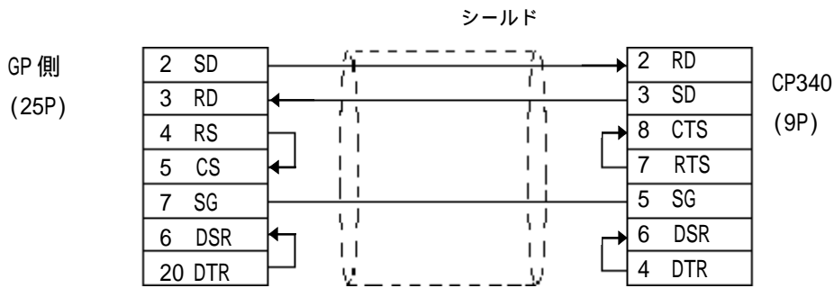
< 結線図 3 > RS-232C
