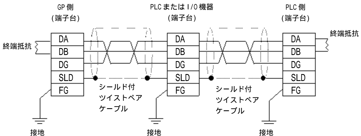
< 結線図 1 > RS-485
