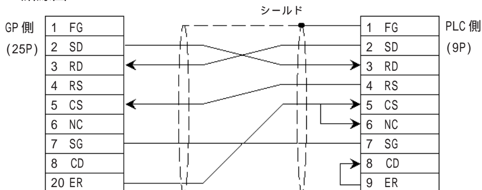
< 結線図 1 > RS-232C
