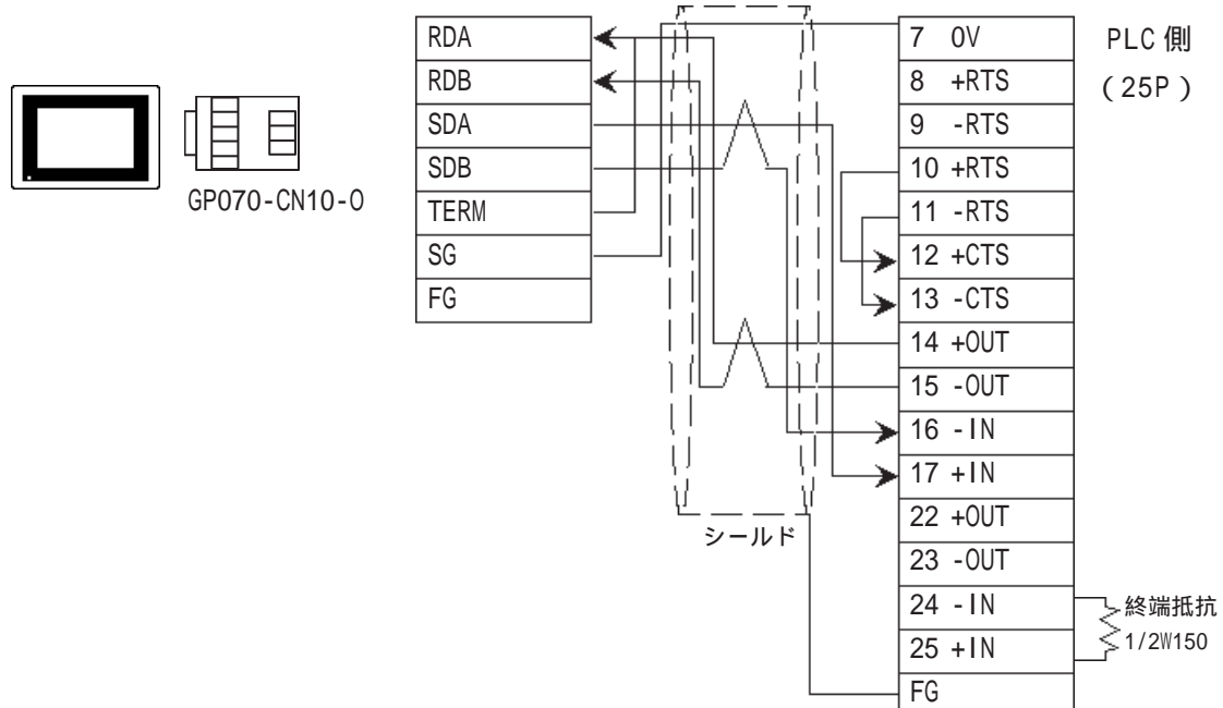
< 結線図 2 > RS-422
