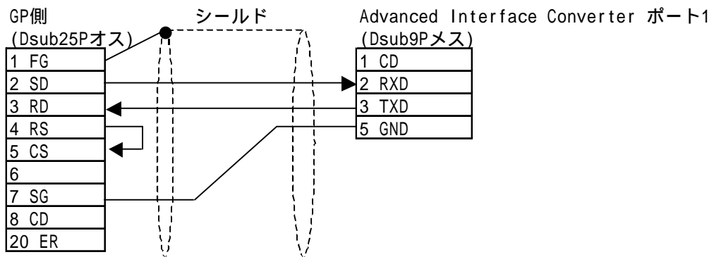
< 結線図 8 > RS-232C
