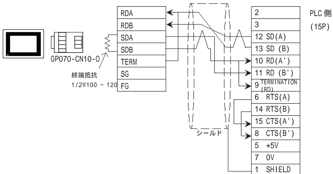
< 結線図 2 > RS-422
