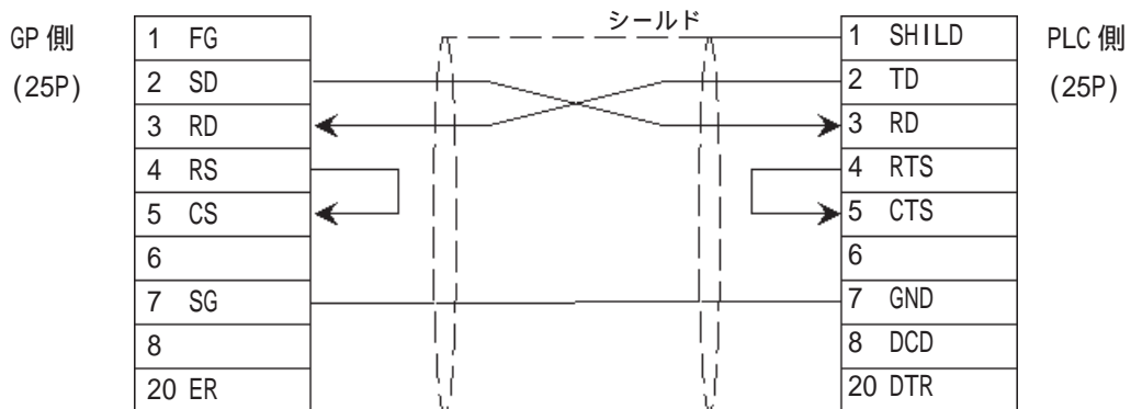
< 結線図 1 > RS-232C
