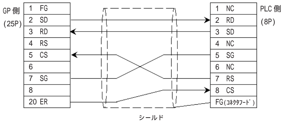
< 結線図 6 > RS-232C
