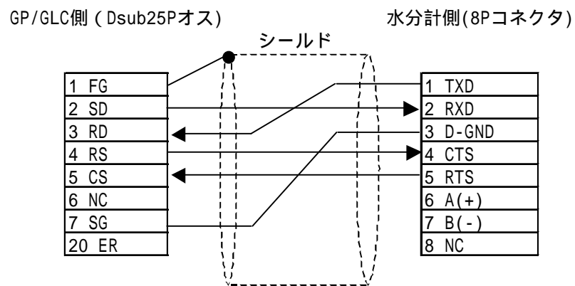
< 結線図 1 > RS-232C
