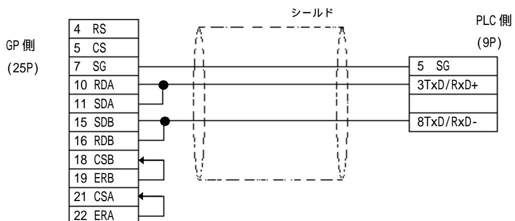
< 結線図 2 > RS-422
