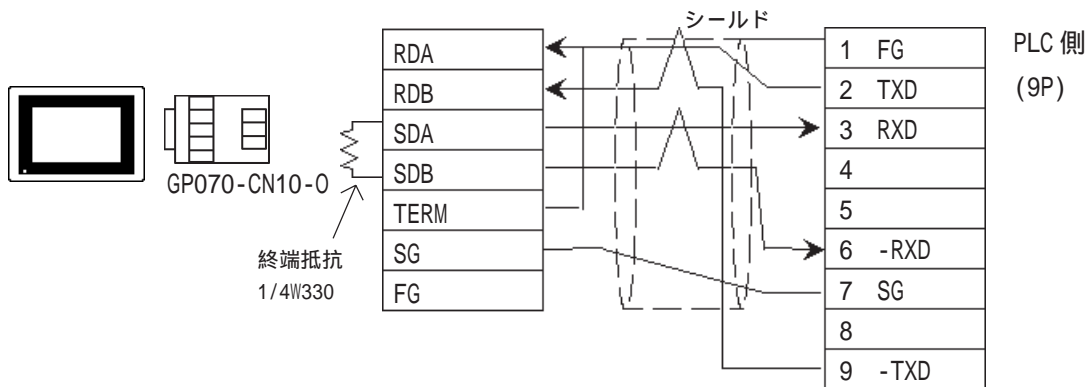
< 結線図 2 > RS-422
