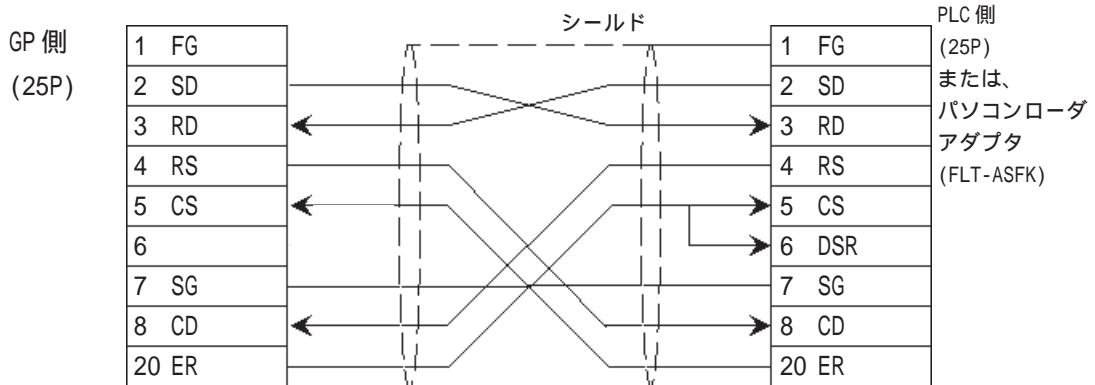
< 結線図 1 > RS-232C
