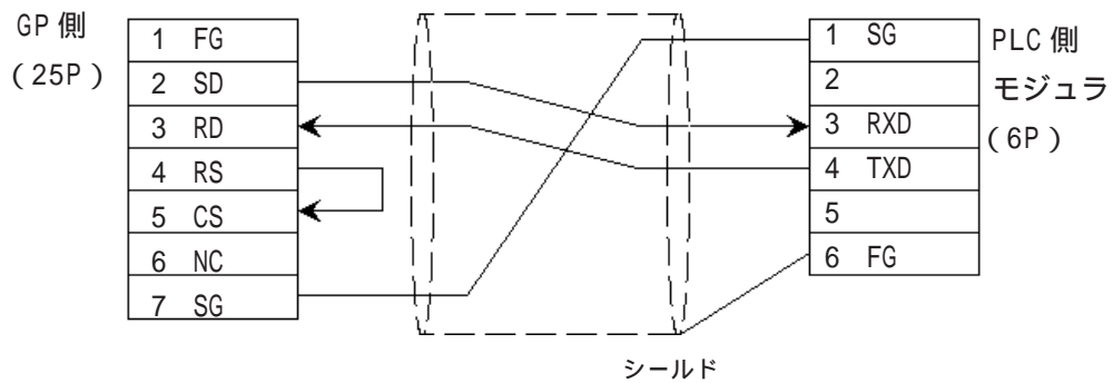
&lt; 結線図 5 &gt; RS-232C
