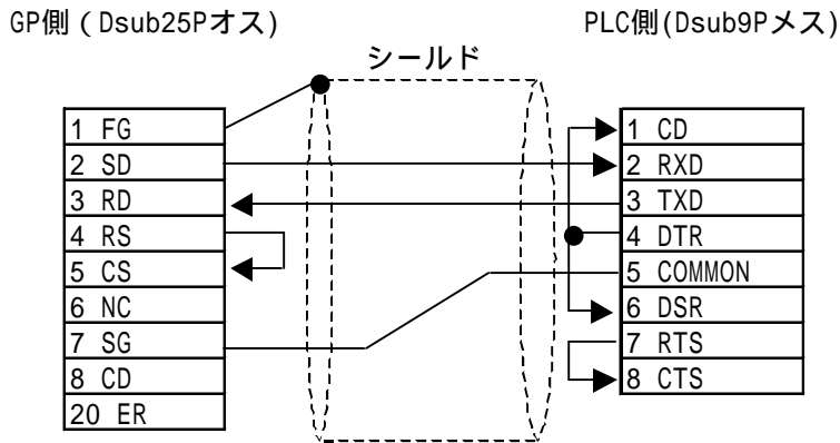
< 結線図 6 > RS-232C
