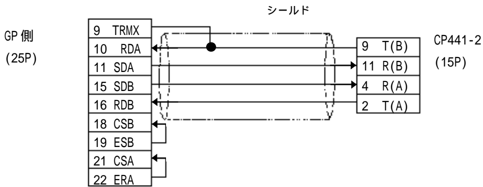
< 結線図 4 > RS-422
