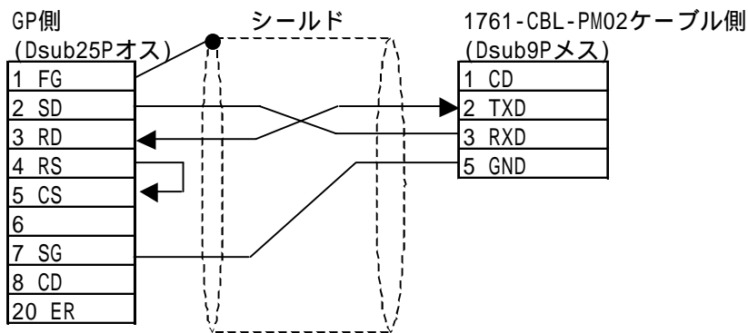
< 結線図 7 > RS-232C
