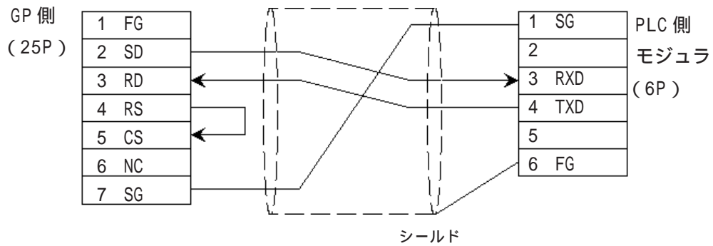
&lt; 結線図 4 &gt; RS-232C
