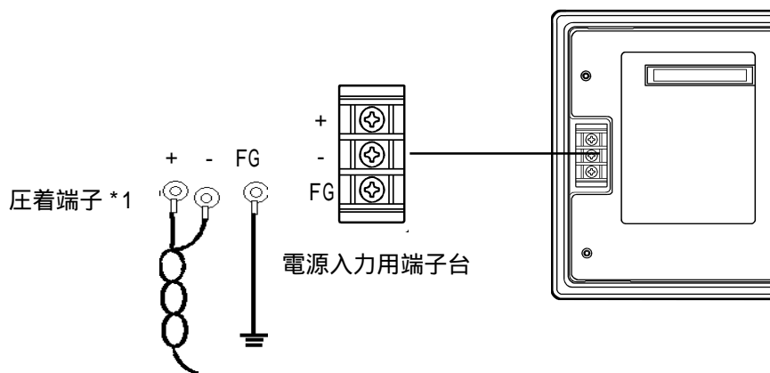
背面図
