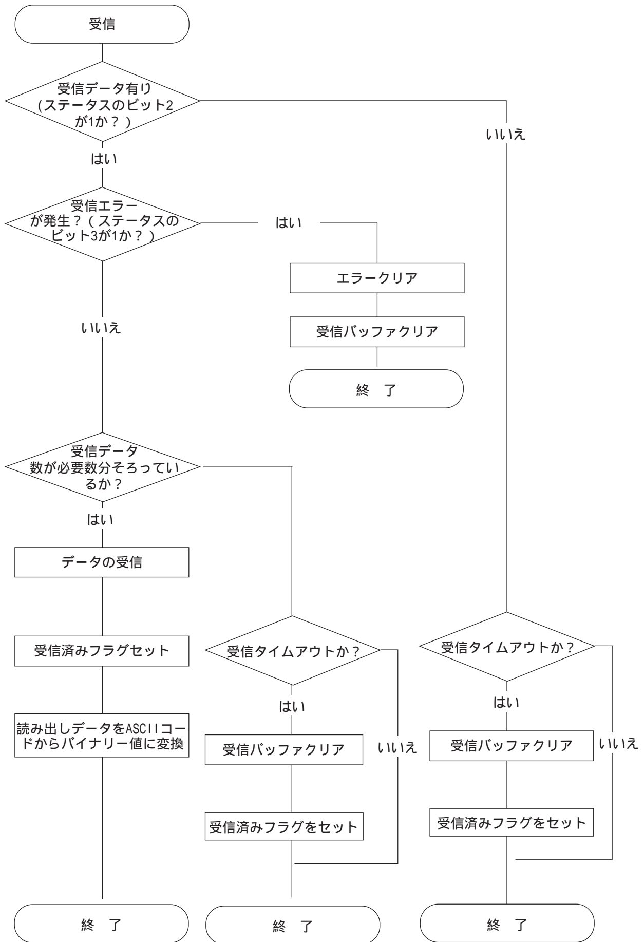
， 受信関数のフローチャート
