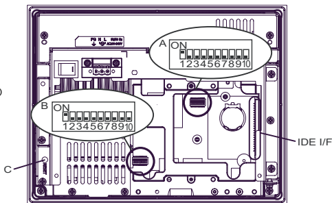
背面内部図 (図は PS3450A-T41)
