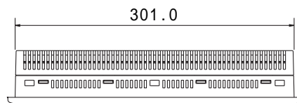
上面図
