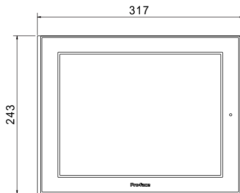
正面図
