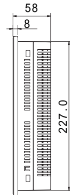
側面図
