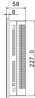
側面図
