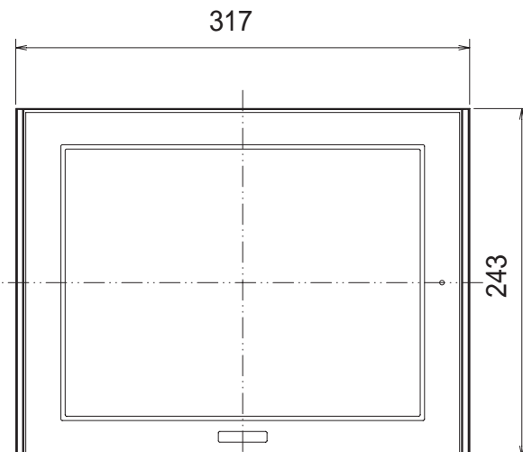
正面圖
