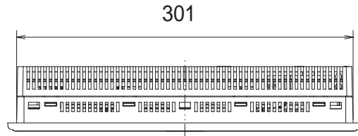
上面圖
