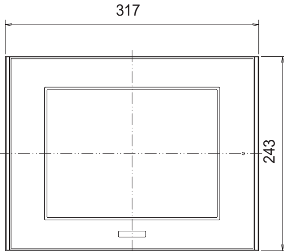
正面圖
