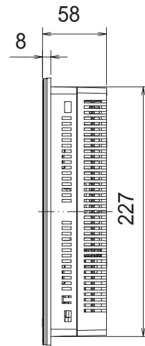
側面圖
