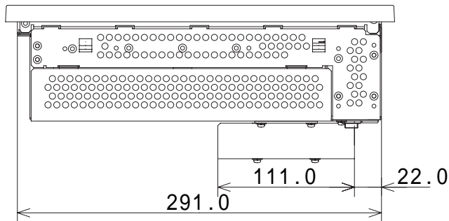
上面図
