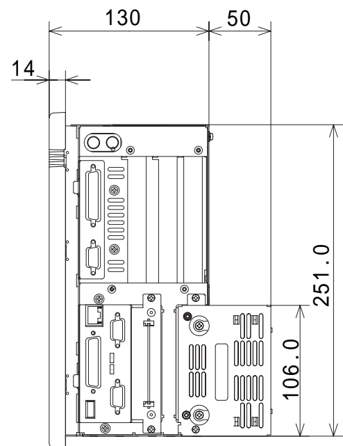
側面図
