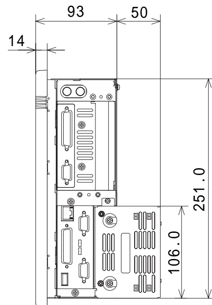
側面図
