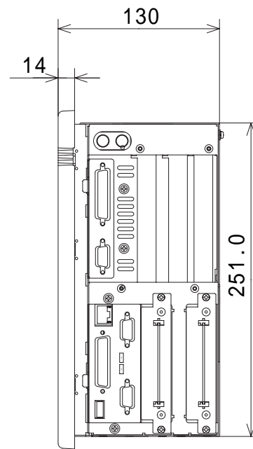
側面図
