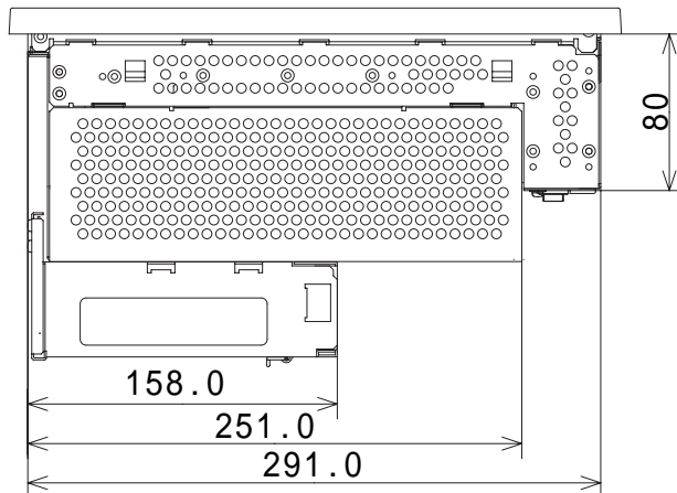
上面図
