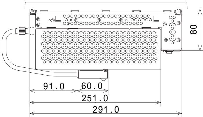
上面図
