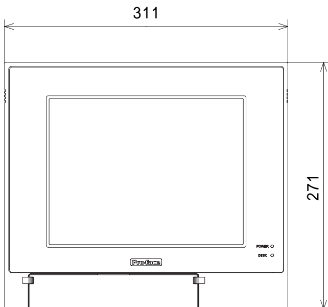
正面図
