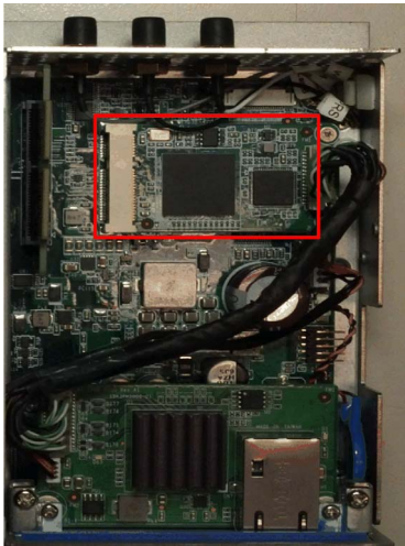
Box Atom:
