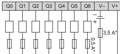
TM221C40U / TM221CE40U
