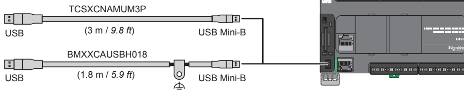
TM221CE●●U
