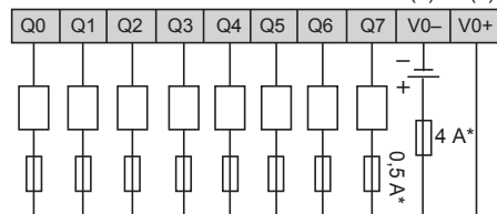
TM221C40U / TM221CE40U
