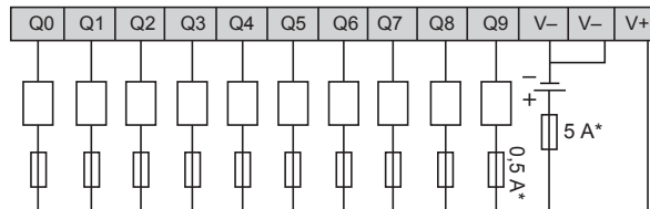
TM221C24U / TM221CE24U
