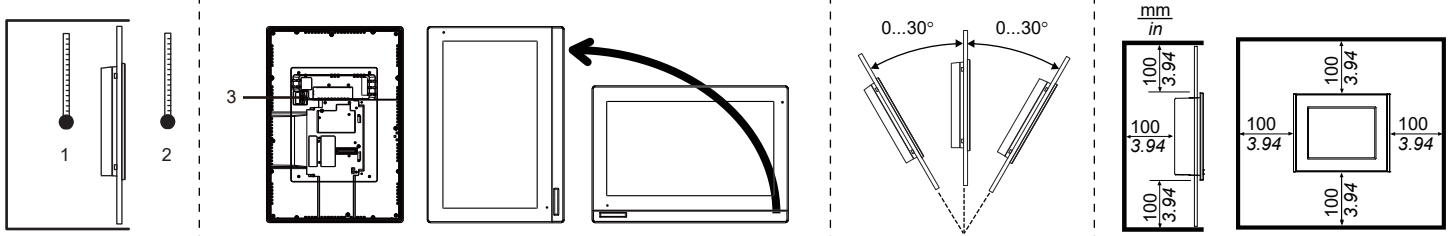
1 Internal temperature/ 盘内温度 /Température interne/Innentemperatur/Temperatura interna/Temperatura interna/ 内部温度 2 External temperature/ 表示面侧温度 /Température externe/Außentemperatur/Temperatura externa/Temperatura esterna/ 外部温度 3 Power connector/ 电源コネクタ /Connecteur d'alimentation/Netzanschluss/Conector de alimentación/Connettore di alimentazione/ 电源接头
