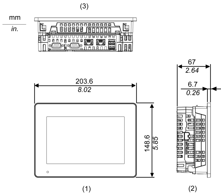
1 正面図
