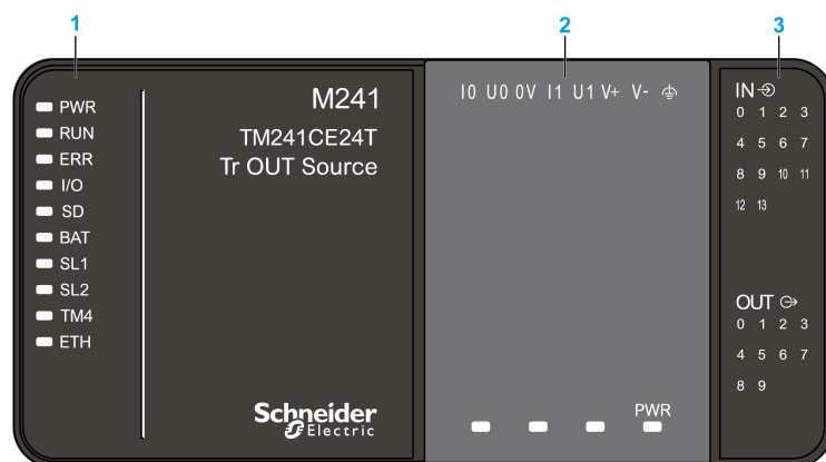
1 システムステータス LED
