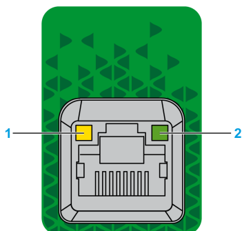
Ethernet ステータス LED
