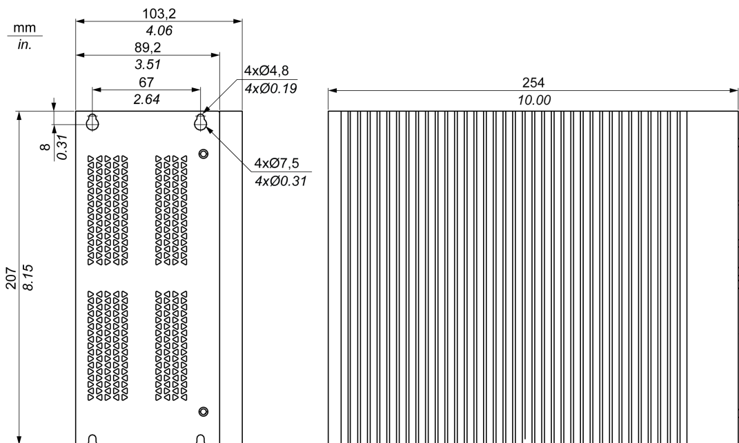
ボックス Celeron/Core i7(2 スロット) の外形寸法 (PFXPU/PFXPP)
