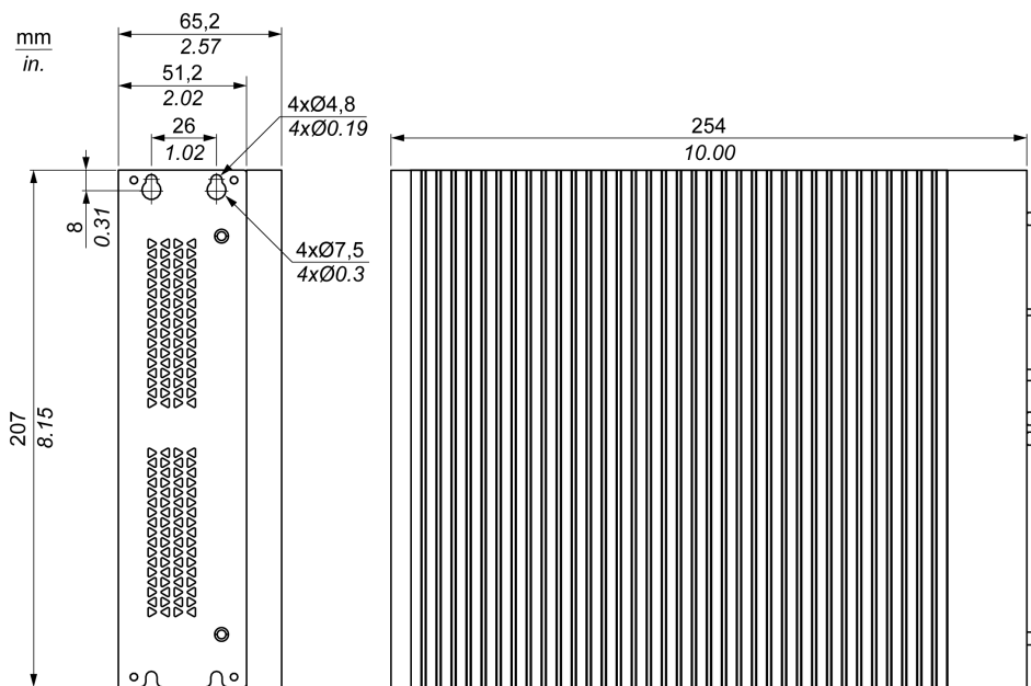
ボックス Celeron/Core i7(0 スロット) の外形寸法 (PFXPU/PFXPP)
