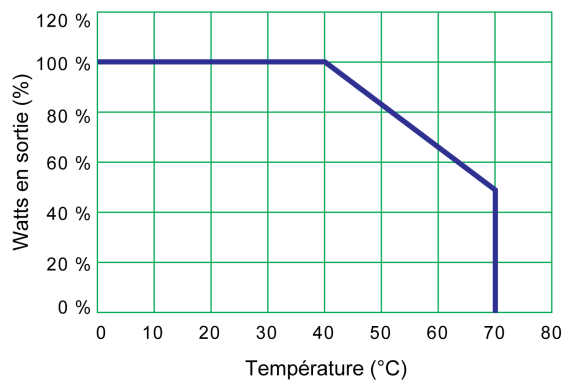
Courbe de réduction de charge de la température de fonctionnement de l'alimentation CA :
