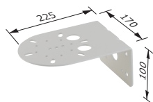
取付L金具 L-1A
