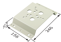
取付M金具 M-2
