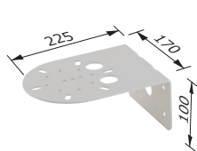
取付L金具 L-1A ¥2,400
