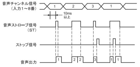
動作モードG タイムチャート
