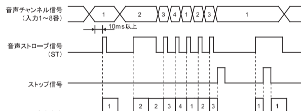
動作モードI タイムチャート
