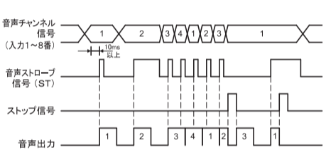
動作モードH タイムチャート
