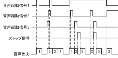
動作モードB タイムチャート
