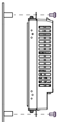
取り付け図 (側面)
