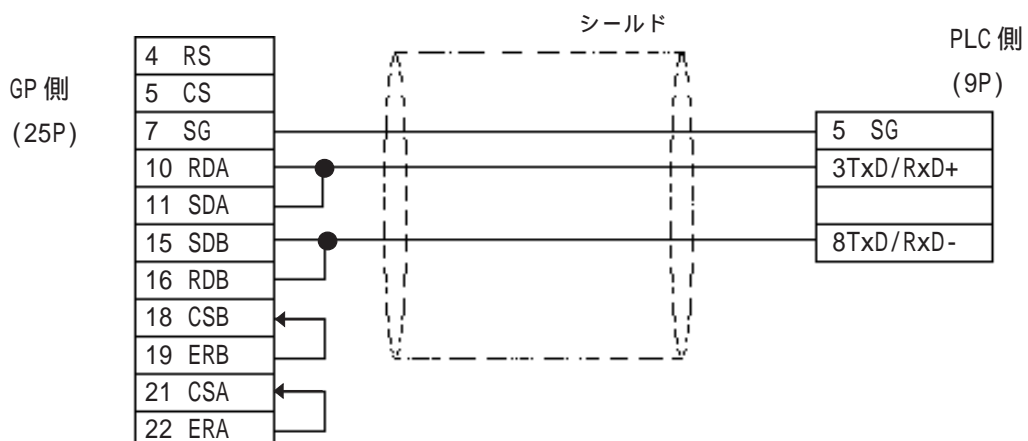
< 結線図 2 > RS-422
