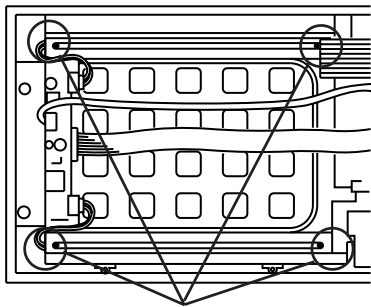
止めネジ
