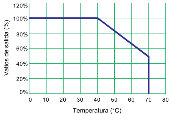
Curva de reducción de la temperatura de funcionamiento de la fuente de alimentación de CA:
