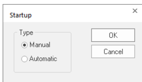
Startup
